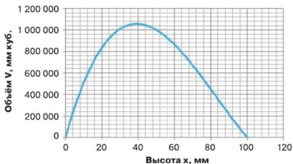
Рис. 3.18. График функции V(x)
