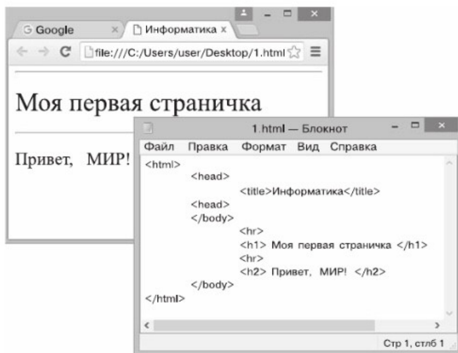
Рис. 4.8. Простейшая веб-страница и её HTML-код
